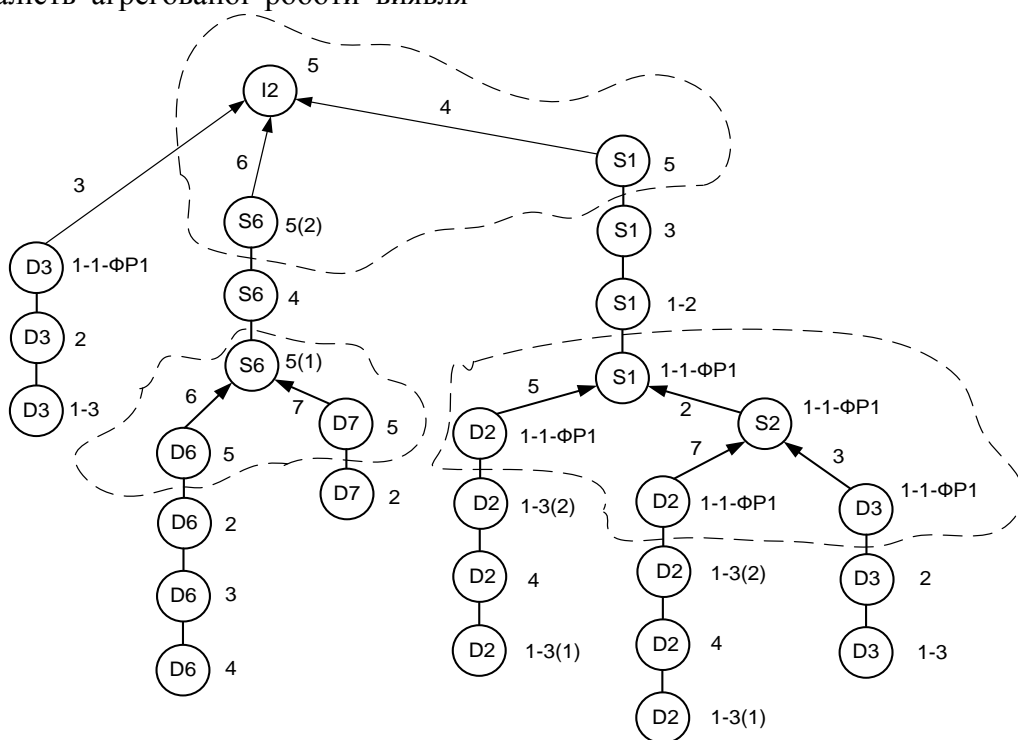
Рис. 2. Приклад вхідного графу виконання робіт та об’єднання в агреговані роботи
